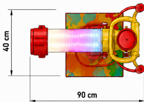
DRAUFSICHT
